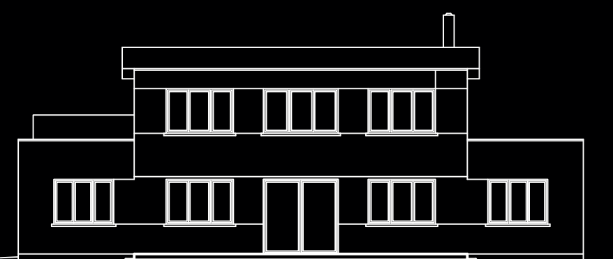
POHLED JIŽNÍ
