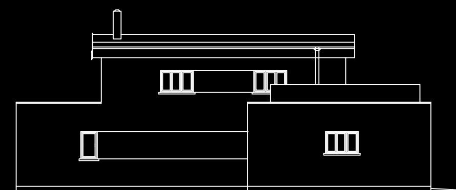
POHLED SEVERNÍ
